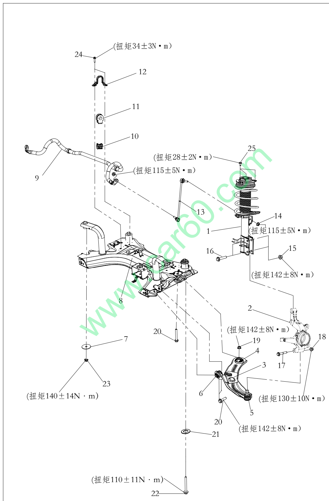
悬架总成零件及装配分解图
